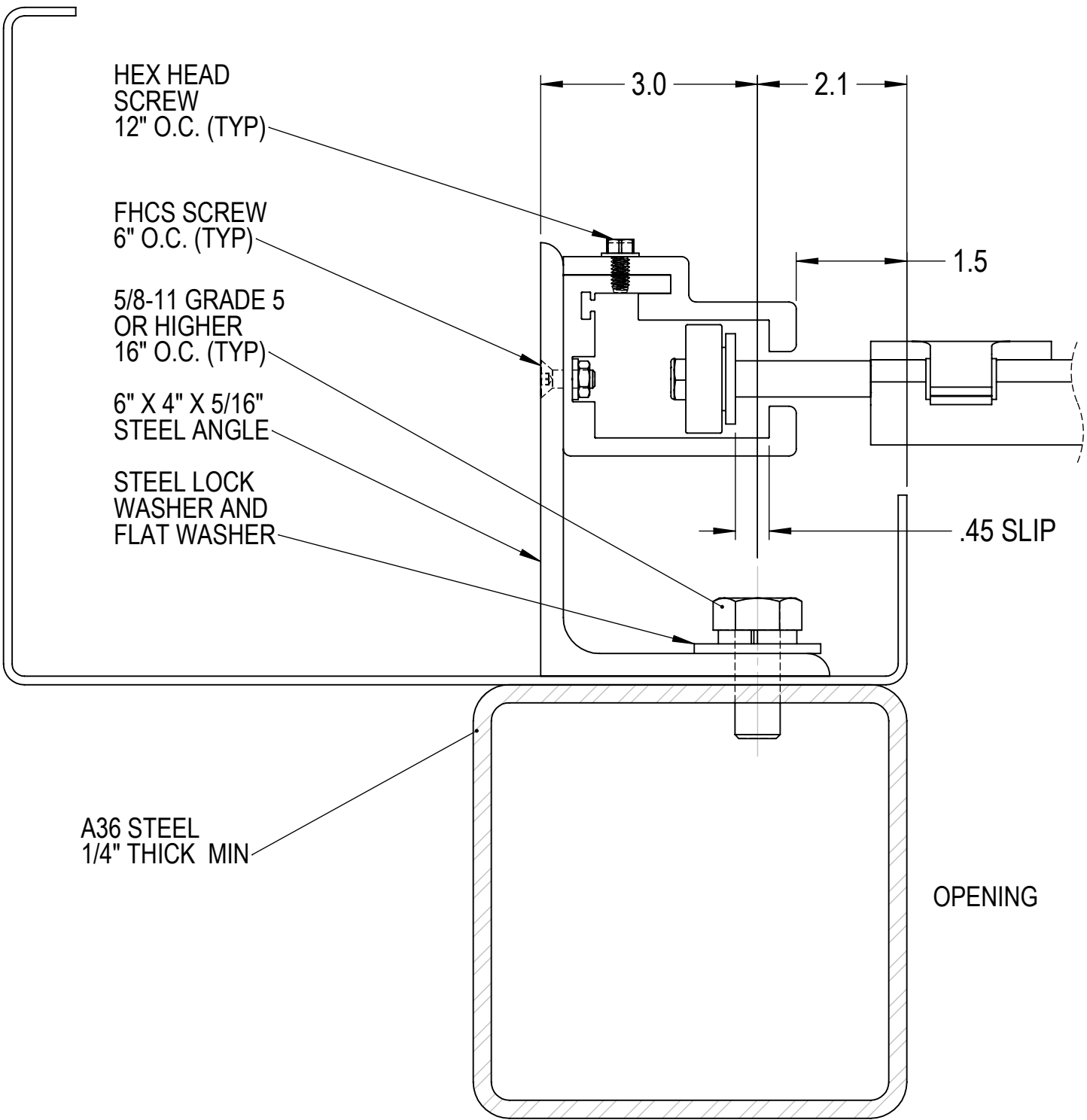
E-GUIDE, STEEL JAMB
